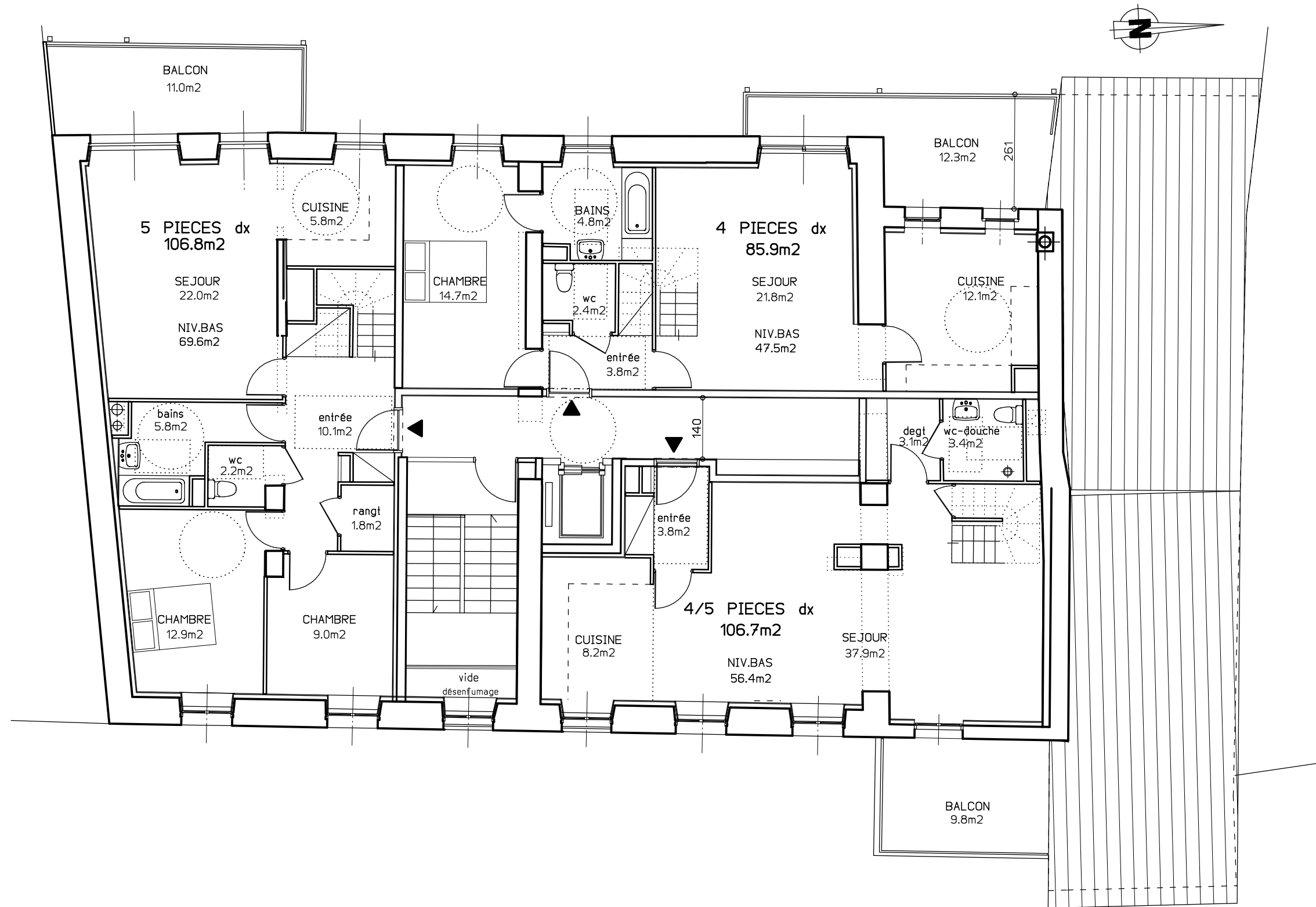
PLAN DU 3° ETAGE
