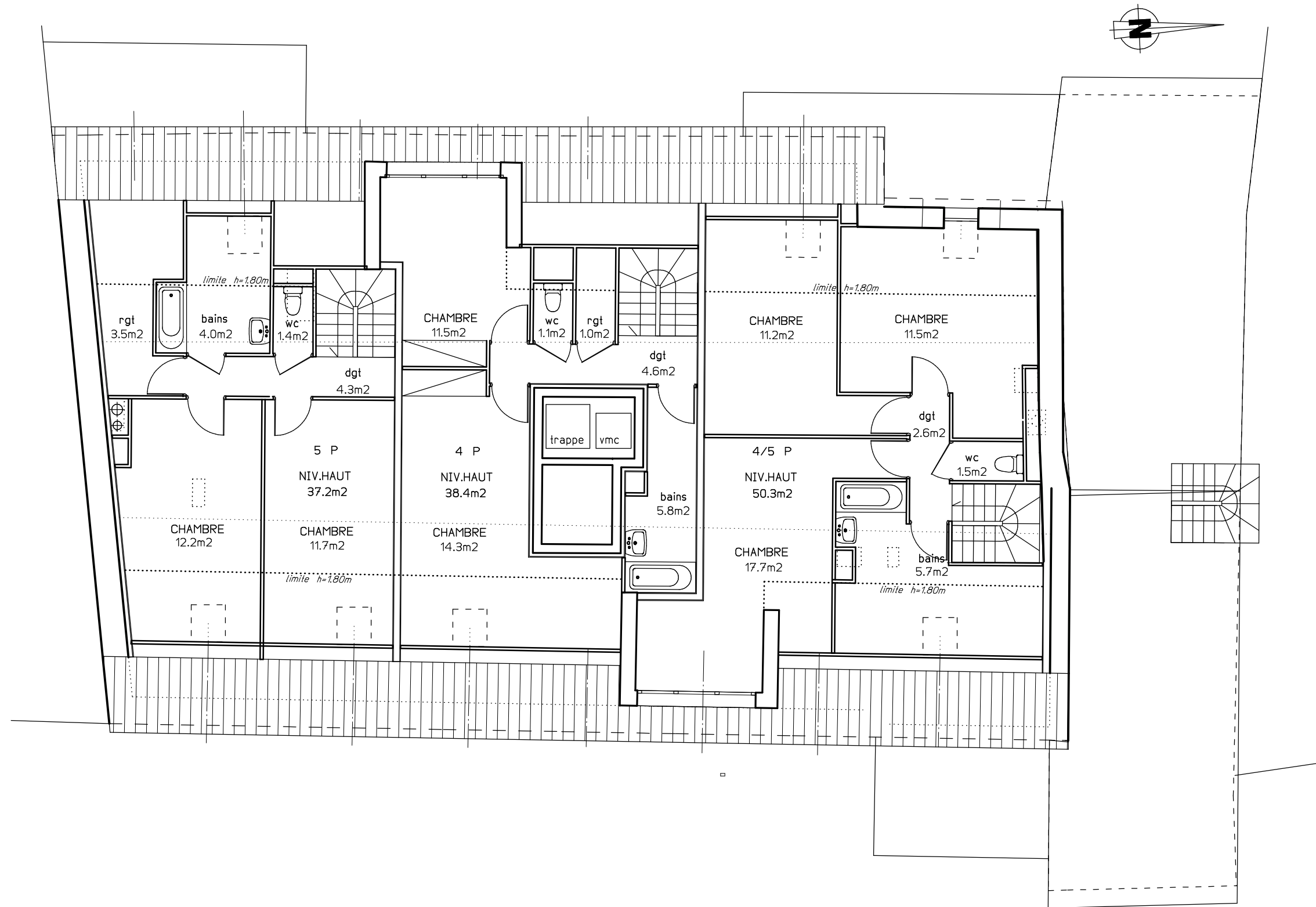
PLAN DES COMBLES
